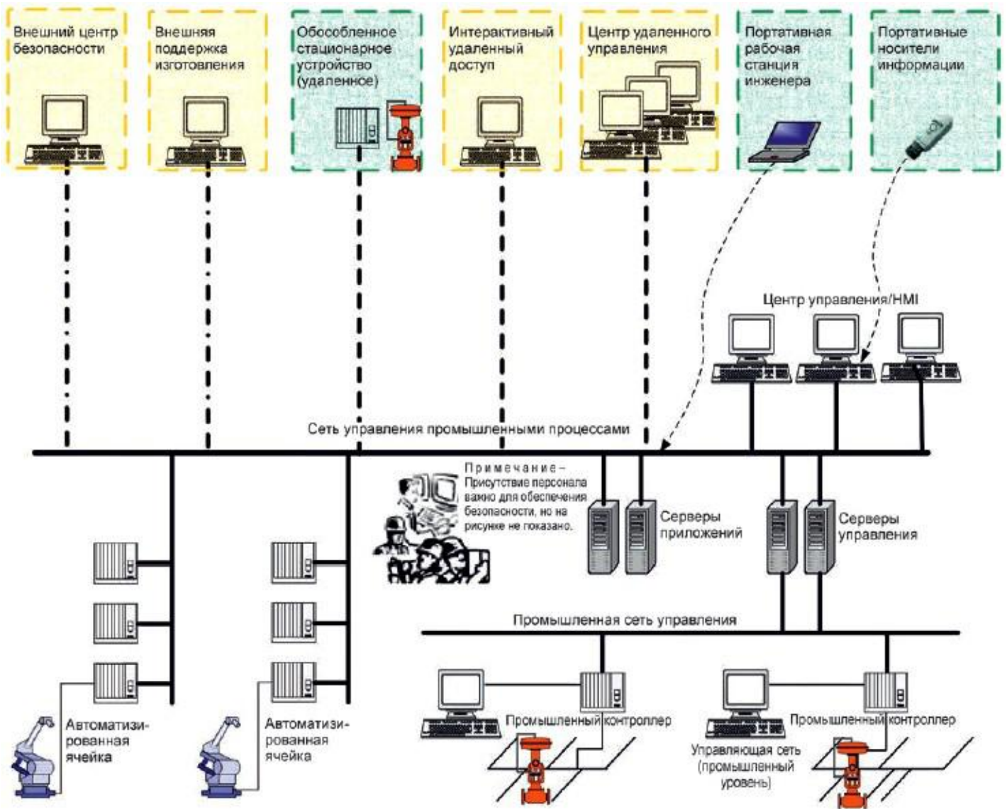
Рисунок 4 - Промышленная система управления (ICS)
