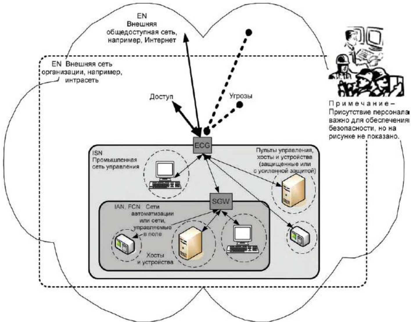
Рисунок 7 - Эшелонированная оборона за счет использования сегментации
