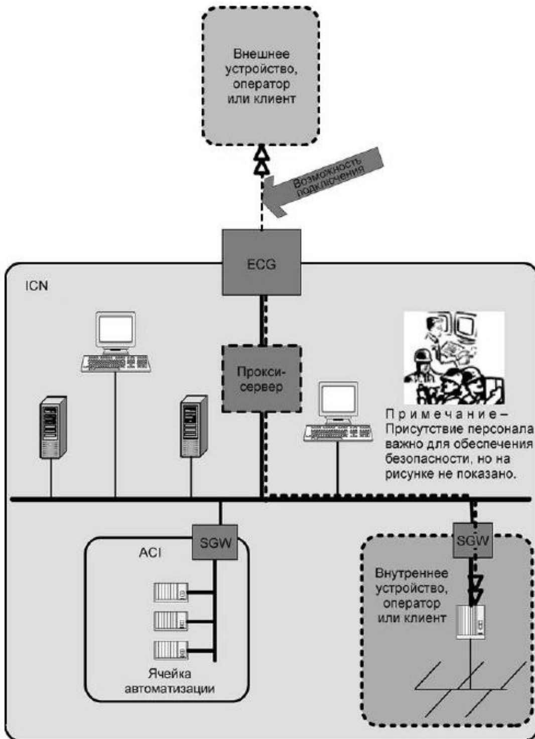
Рисунок 9 - Общие внешние соединения
