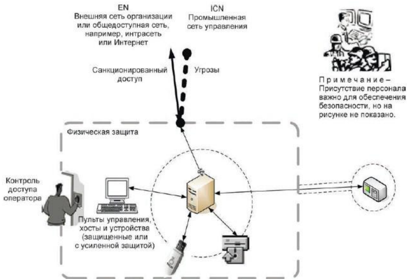
Рисунок 6 - Защита устройства - усиление защиты и управление доступом
