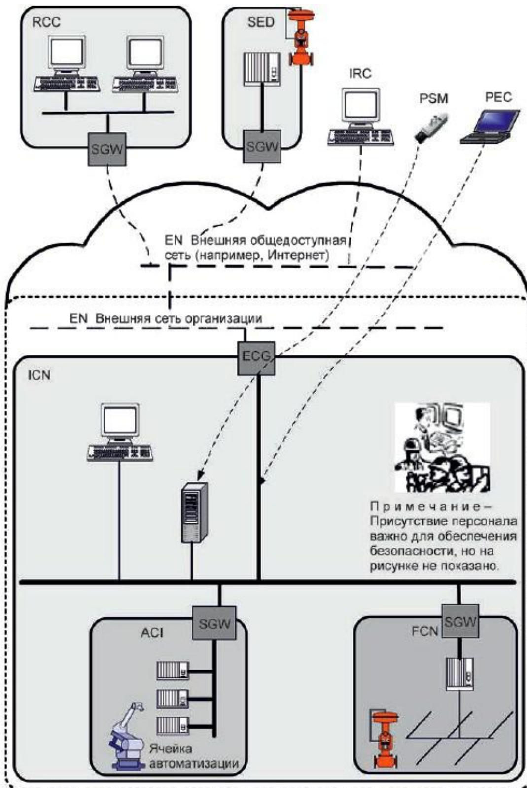
Рисунок 8 - Пример - сегментация ICS
