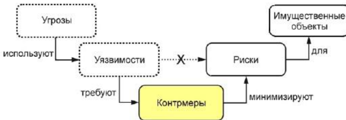
Рисунок 1 - Взаимосвязь угроз-рисков
